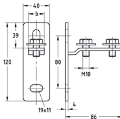
MPC-Stirnflansch, quer
