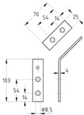
Montagewinkel 45°
