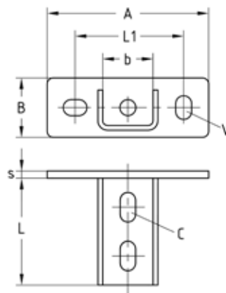
MPC-Sattelflansch, quer
