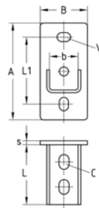
MPC-Sattelflansch, längs
