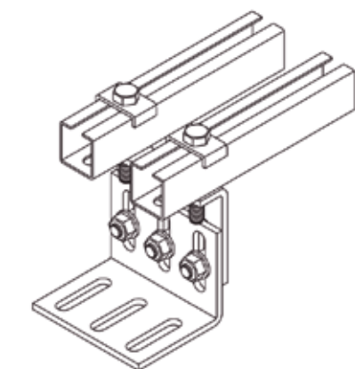
In hoogte verstelbare onderconstructie voor vastpunten en glijbevestigingen
