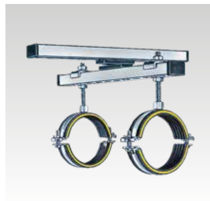
Schiebebefestigung für Schiebewege in rohraxialer und radialer Richtung
