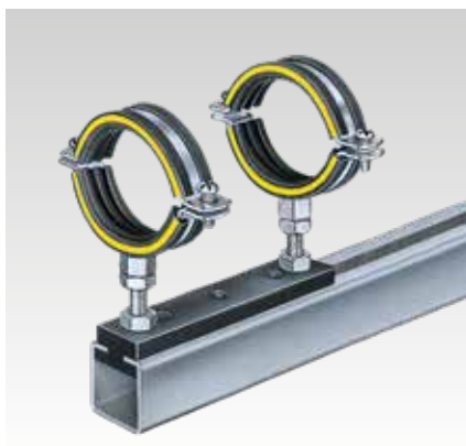
Gleitkörper M10 als stehende Befestigung
