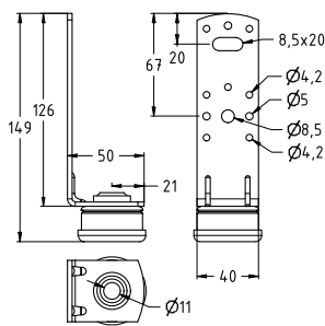
Luftkanalwinkel Typ III
