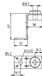
Luftkanaldoppelwinkel Typ I
