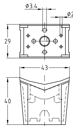
Universalhalter
